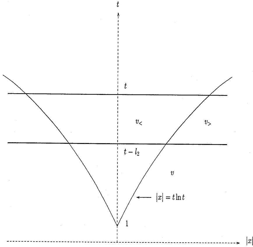
Fig. 12.1 Partage de la région d'intégration dans le Lemme 12.5 .
