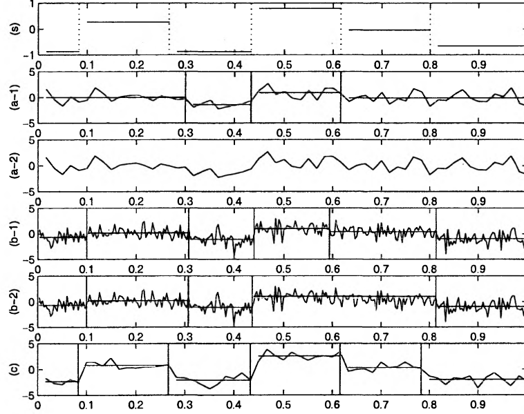
FIG. 4.11: Graphiques des estimateurs pénalisés obtenus par la méthode calibrée (a – 1), (b – 1) et (c), et ceux obtenus par la méthode de sélection de modèle à variance connue et estimée (a – 2), (b – 2) et (c), pour les trois réalisations.
