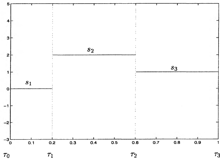
FIG. 2.1: Représentation de la fonction s .
