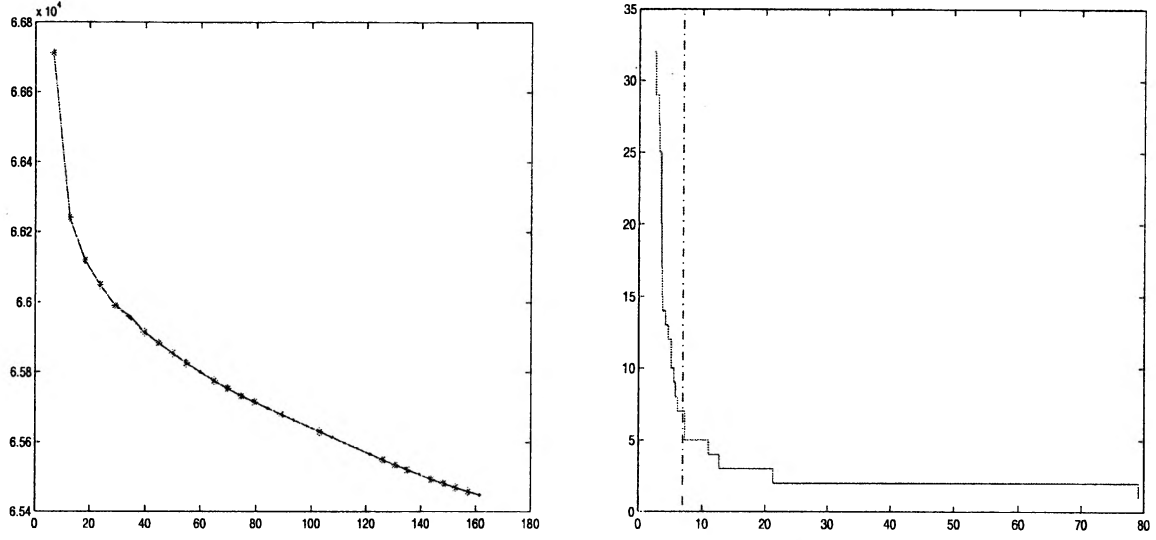
FIG. 7.8: (f_n(D), \gamma_n(\hat{s}_D)) pour D = 1, \dots, 32 (à gauche) et \sum_{i=1}^K D_i 1_{[\alpha_i, \alpha_{i+1}[} (à droite) où le symbole -. correspond à 2\hat{\alpha} .
