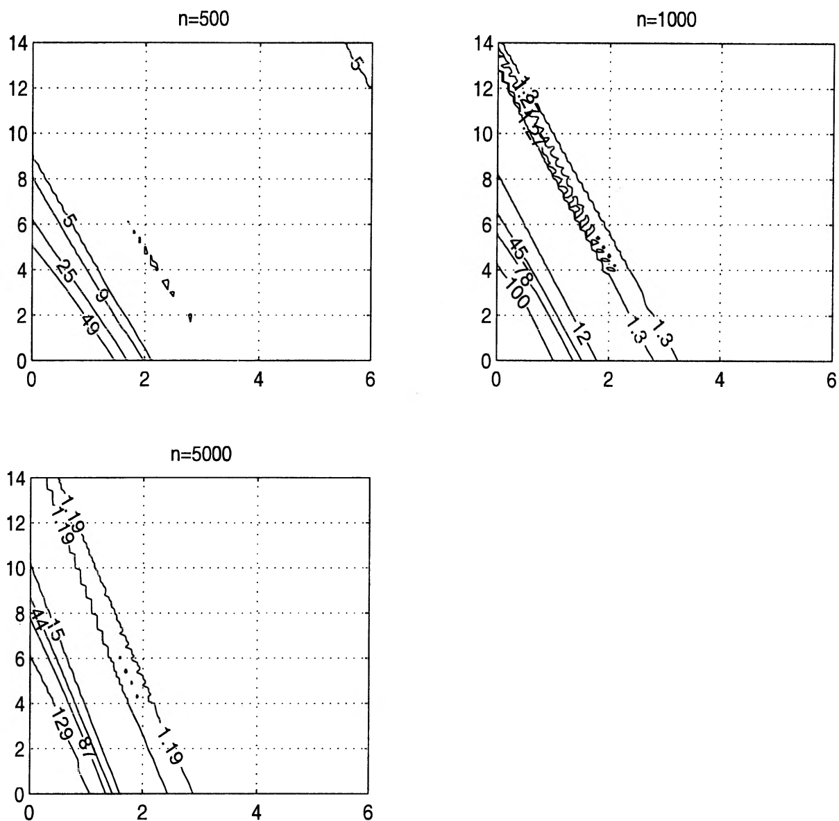
FIG. 3.5: Graphe de la fonction (c_1, c_2) \rightarrow F_n(c_1, c_2) pour n = 500, 1000, 5000 .
