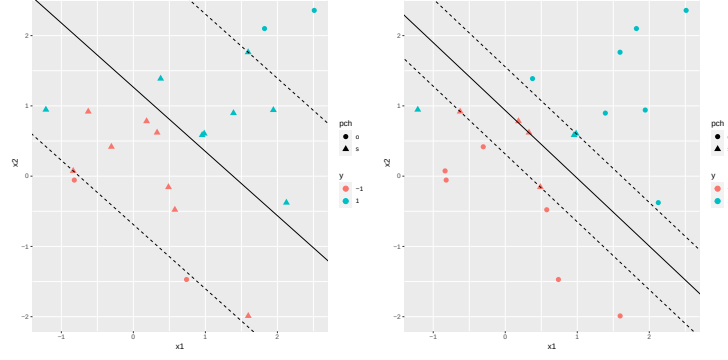
FIGURE 13.3 – Deux plans séparateurs : défini avec une grande marge (à gauche, et donc de nombreux points supports) ou une faible marge (à droite, peu de points supports). Les points supports sont les observations qui sont situés dans la zone d'indécision, entre les deux droites en pointillés ou les points mal classés hors de la zone d'indécision.
