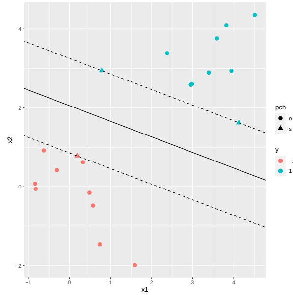
FIGURE 13.2 – Représentation du séparateur linéaire à marge rigide (trait noir plein), et des points supports (triangles). La marge est la distance entre les deux droites pointillées.
