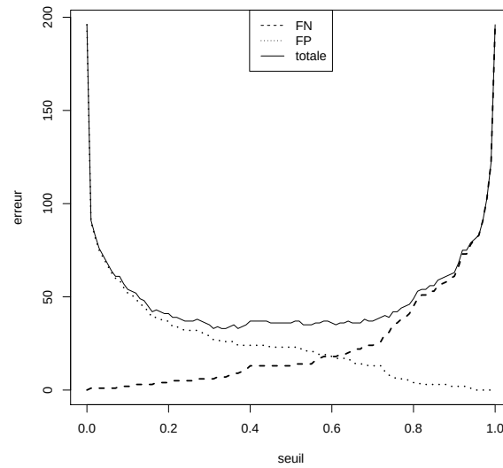
FIGURE 10.1 – Evolution des erreurs en fonction du seuil (exprimé dans l'échelle de la probabilité)
