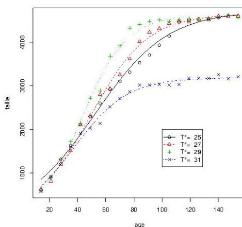
FIGURE 7.2 – Régression non linéaire : Croissance des alevins en fonction de la température de l'eau
