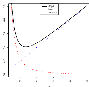
FIGURE 11.1 – Compromis Biais-Variance : avec peu de paramètres, le biais est important. Il diminue avec le nombre de paramètres alors que la variance augmente. L'EQM réalise un compromis entre les deux.
