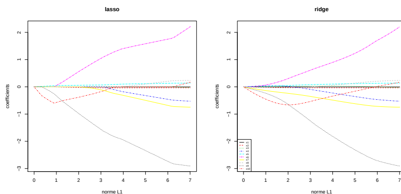
FIGURE 12.1 – Régression lasso et ridge sur un exemple
