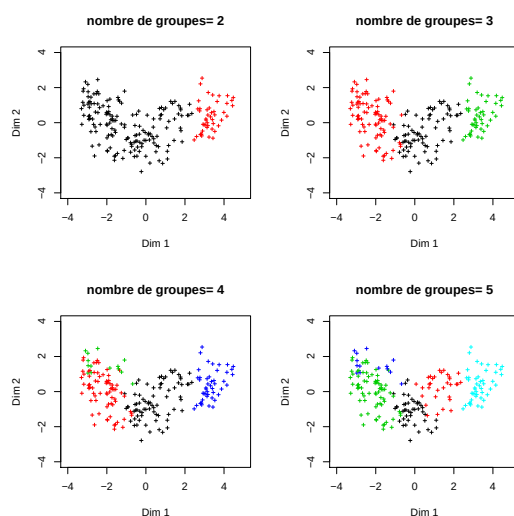
FIGURE 6.3 – Les groupes sélectionnés suivant la CAH suivant le premier plan principal
