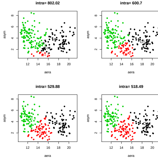
FIGURE 6.1 – Différentes étapes de l'algorithme des K -moyennes ( K=3 ) représentées sur le premier plan principal
