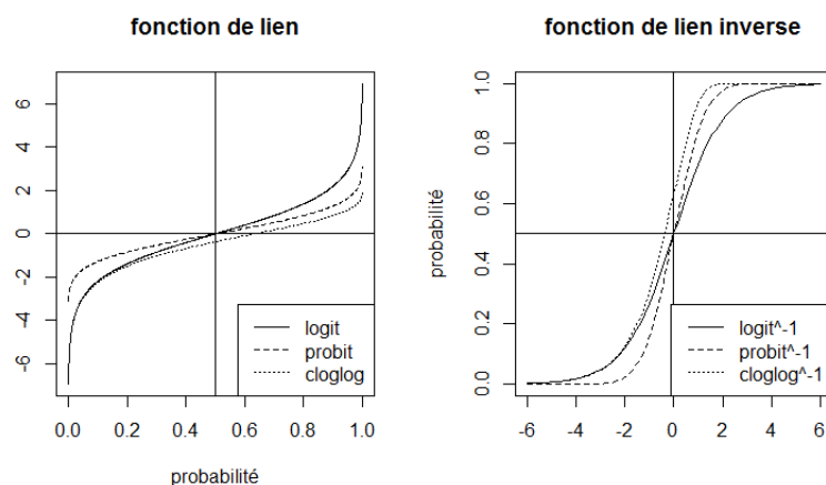
FIGURE 9.1 – Quelques exemples de fonctions de lien et leur inverse
