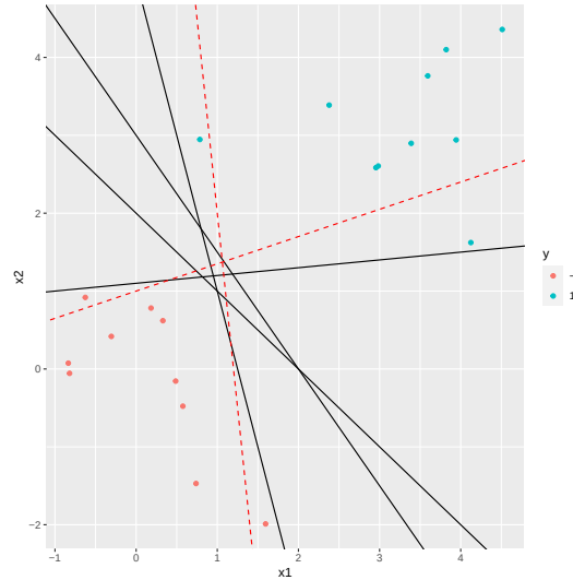
FIGURE 13.1 – Les droites sont des hyperplans de \mathbb{R}^2 , les noires sont séparatrices des points rouges et bleus
