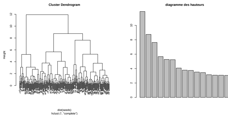
FIGURE 6.2 – Dendrogramme et diagramme en barre des indices d'agrégation
