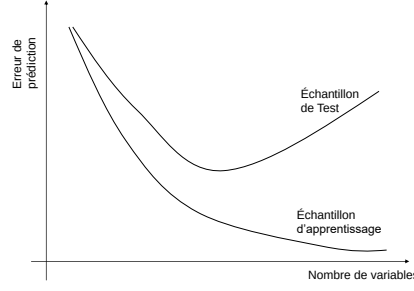
FIGURE 11.2 – Biais de la somme des carrés résiduels calculée sur l'échantillon d'apprentissage pour estimer le risque. L'estimation sur un échantillon test n'est pas biaisée.
