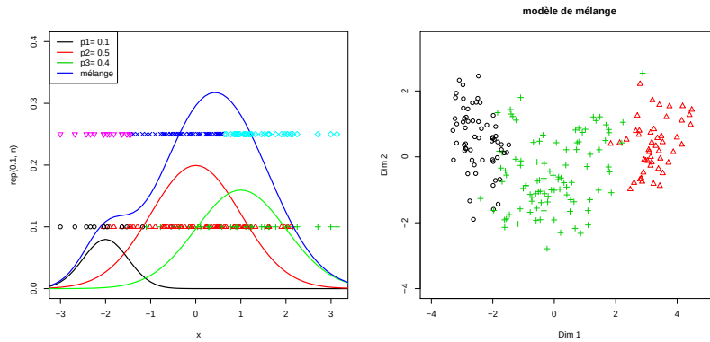
FIGURE 6.5 – L'allocation des observations suivant la règle du MAP : à gauche, dans le cadre d'un mélange univarié, les affectations sont matérialisées par des points alignés sur la ligne du haut ; à droite, dans le cas d'un mélange multivarié appliqué aux données seeds, les groupes sont représentés par différentes couleurs sur le premier plan principal.
