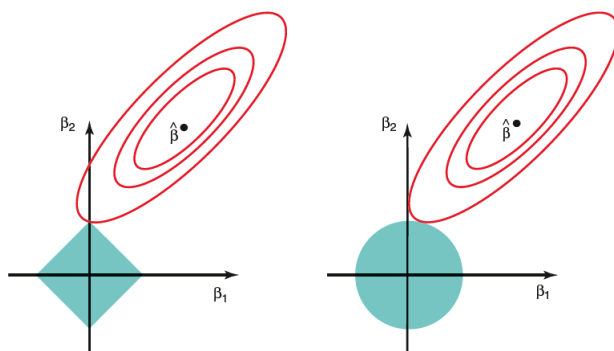
FIGURE 12.2 – Régression lasso (à gauche) et ridge (à droite)
