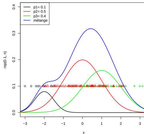
FIGURE 6.4 – Loi de mélange de trois gaussiennes univariées
