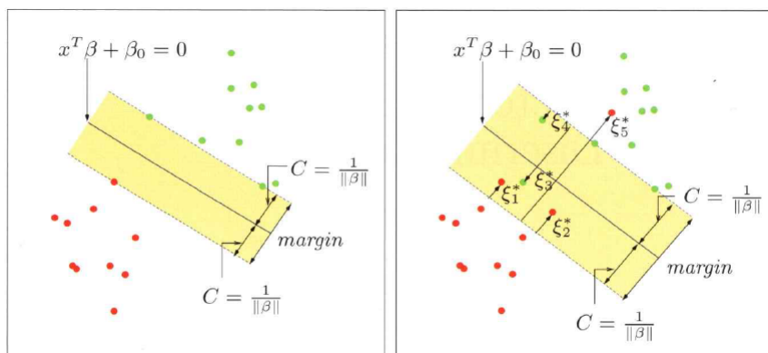
FIGURE 13.4 – A gauche, cas SVM à marge dure : il existe un hyperplan séparateur et les vecteurs supports sont à la frontière de la zone d'indécision. A droite, cas SVM à marge souple : il n'existe pas d'hyperplan séparateur ; les vecteurs supports sont les observations à l'intérieur de la zone d'indécision, qu'elles soient mal classées (observation associée à la variable \xi_3^* ) ou bien classées (observations associées aux variables \xi_1^*, \xi_2^*, \xi_4^* ) d'une part, les observations mal classées à l'extérieur de la zone d'indécision (observation associée à la variable \xi_5^* ) d'autre part. Figure issue de Hastie et al. (2001)
