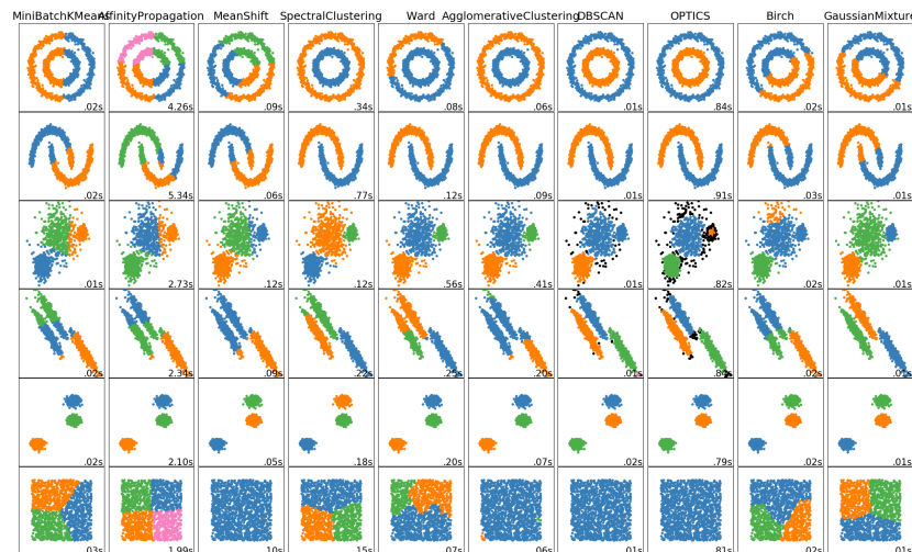
FIGURE 6.6 – Comparaison de différentes méthodes de clustering, package scikit-learn de Python, https://scikit-learn.org/stable/modules/clustering.html
