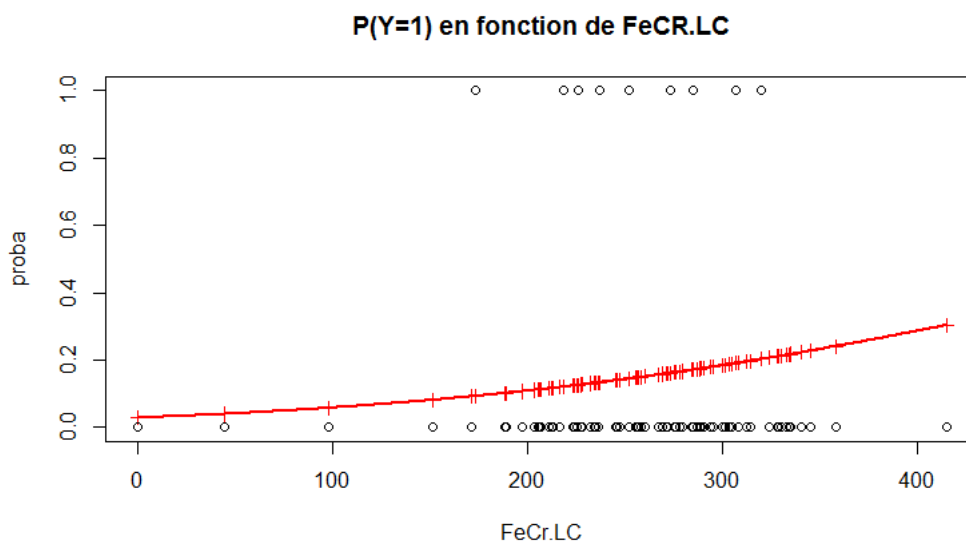
FIGURE 9.3 – Taux de pièces défectueuses en fonction de la concentration de FeCr.LC
