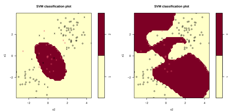
FIGURE 13.5 – Influence du coût \gamma sur les résultats (à paramètre du noyau constant)
