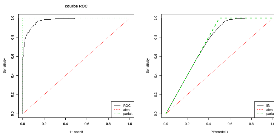
FIGURE 9.2 – Exemple de courbe ROC (à gauche) et de lift (à droite)
