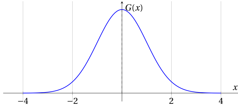
FIGURE 7.1 – Courbe de la fonction densité de la loi de Gauss.
