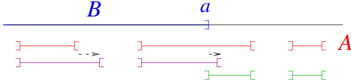
FIGURE 4.2 – Représentation schématique des intervalles ]a_i, b_i[ (rouge) recouvrant A , et de leurs troncations recouvrant A \cap B (famille \mathcal{F}_1 , violet) et A \cap B^c (famille \mathcal{F}_2 , vert). Le prolongement par \epsilon 2^{-i} est indiqué par une flèche.
