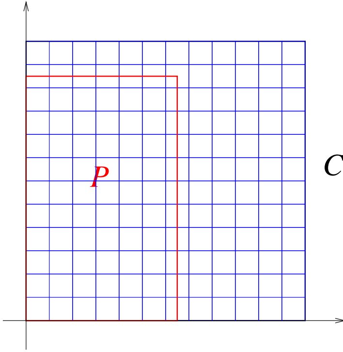
FIGURE 4.5 – Partition de l’hypercube unité C en n^d « petits cubes » P^{(k)} , permettant d’approcher un pavé P .
