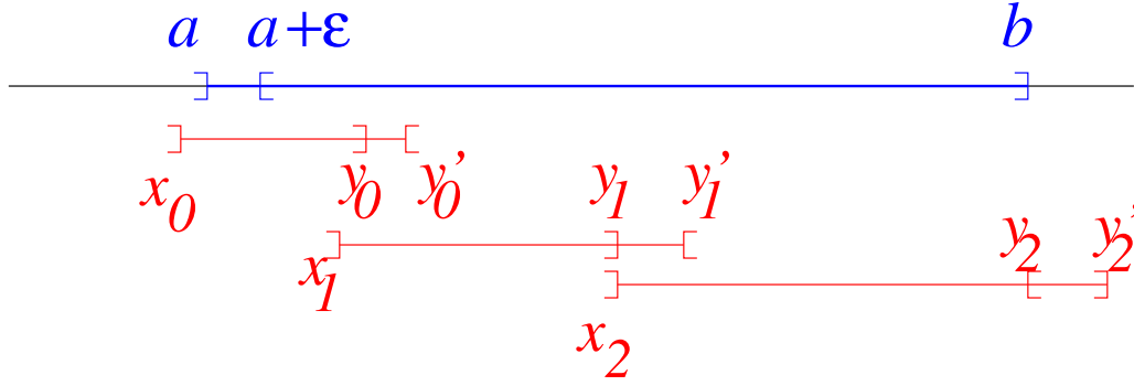
FIGURE 4.7 – Intervalles intervenant dans la preuve de l'inégalité F(b) - F(a) \leq \sum_{i=0}^{\infty} (F(y_i) - F(x_i)) .
